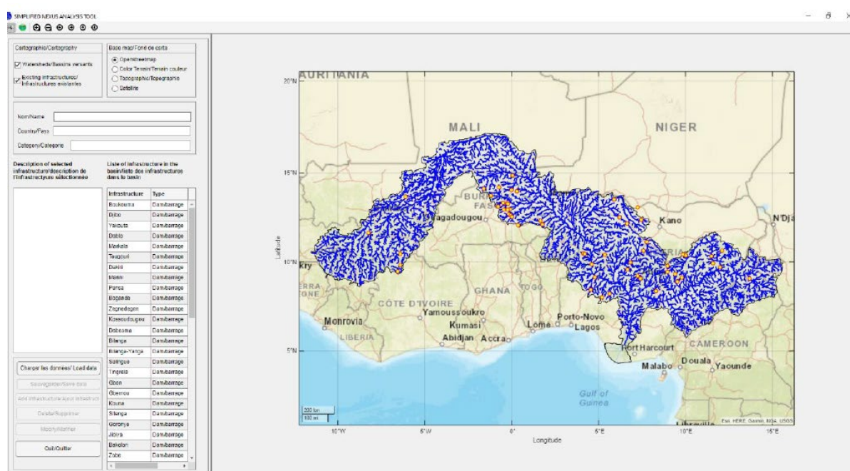
Figure 3.4.3.3.1. : Vue de l'interface de l'outil avec les réseaux hydrographiques et les ouvrages de mobilisation des eaux du bassin 21
